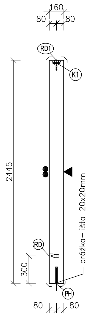
ŘEZ A-A
